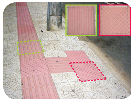
Na foto, podemos ver um exemplo da aplicação dos pisos táteis em uma calçada: o piso direcional, que indica a direção a seguir, e piso alerta, que aponta a mudança de direção e presença de desnível (rampa).
