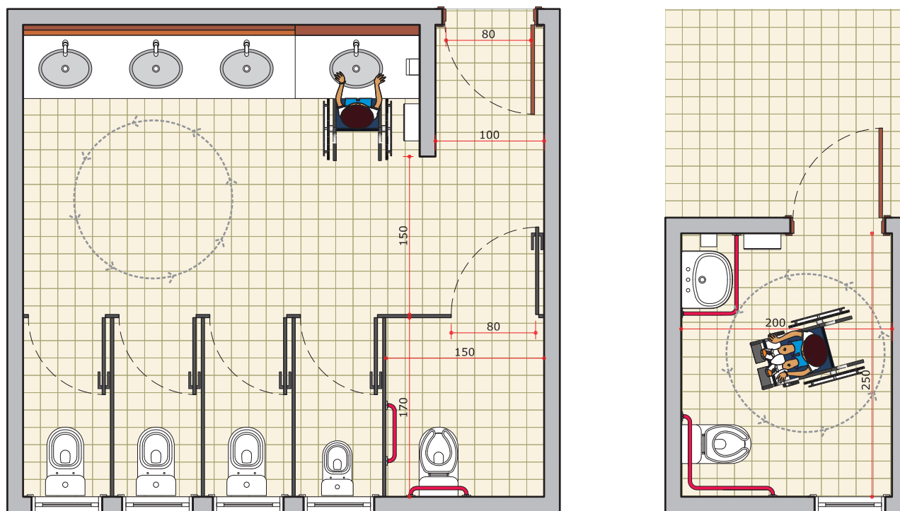
Na desenho da esquerda, exemplo de reforma de sanitário existente, e no desenho a direita, exemplo de novo banheiro.
