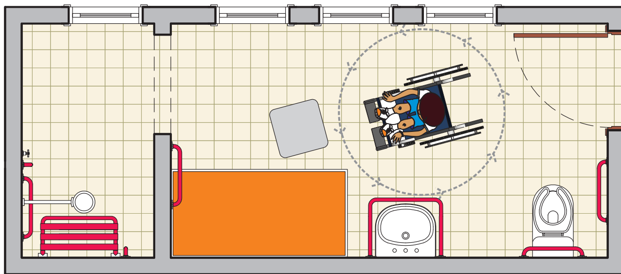
Planta baixa ilustrando exemplo de trocador conforme descrição da opção 2
